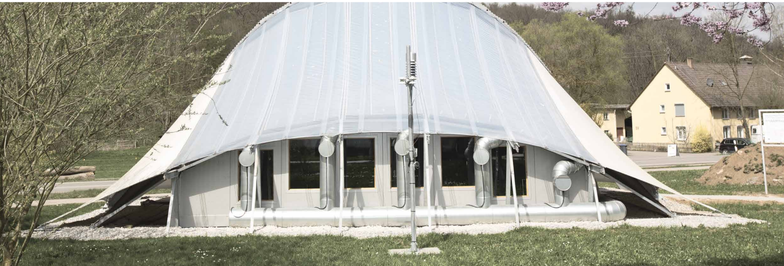
Eisbärvavillon: textiler Membranbau mit höchster Energieeffizienz und verlustfreiem Wärmespeicher
