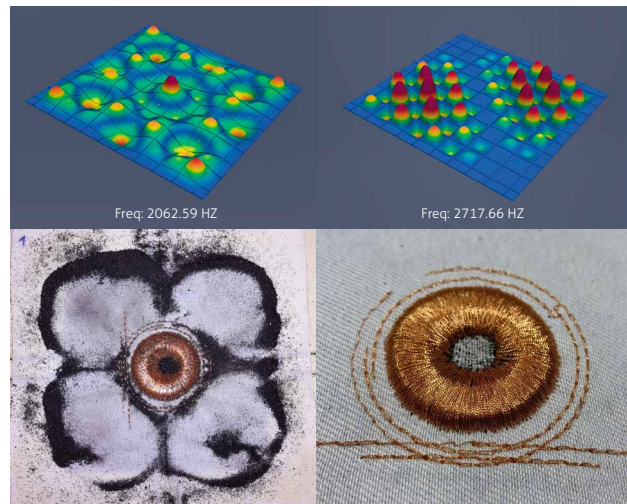
Oben: Eigenmoden lokal-resonanter Textilien
