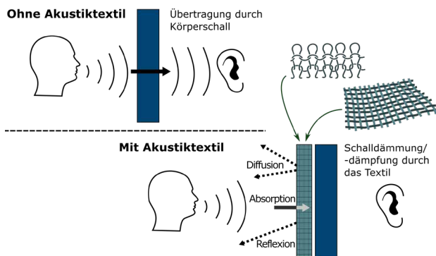
Prinzipische Skizze der Übertragungsminderung durch ein textiles Dämmsystem
